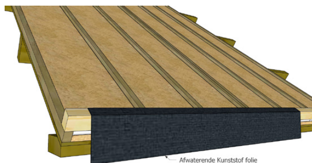
Figuur 6 - Afwaterende kunststof folie
