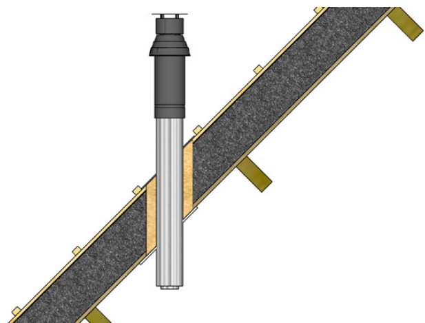
Figuur 13 - Detail sparing mantelbuis
