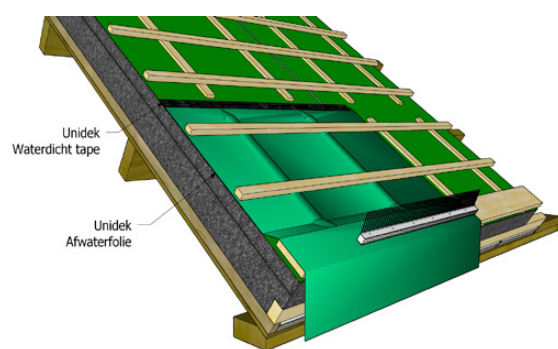
Figuur 1 - Detail gootafwatering met Unidek Afwaterfolie en Unidek Waterdicht tape
