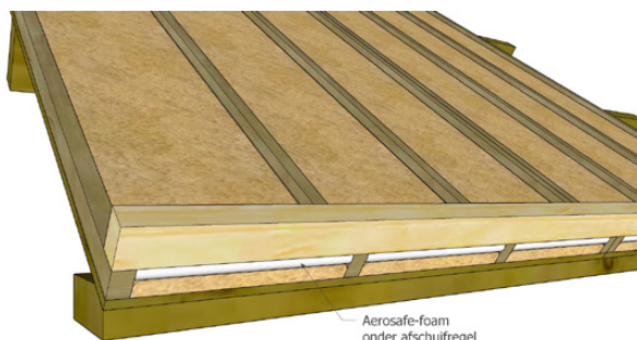
Figuur 5 - Aerosafe-foam onder afschuifregel
