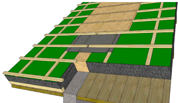
Figuur 12 - Detail woningscheidende wand
