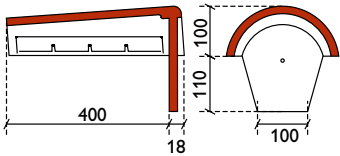
uni-beginvorst
