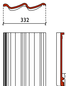
dubbele welpan
